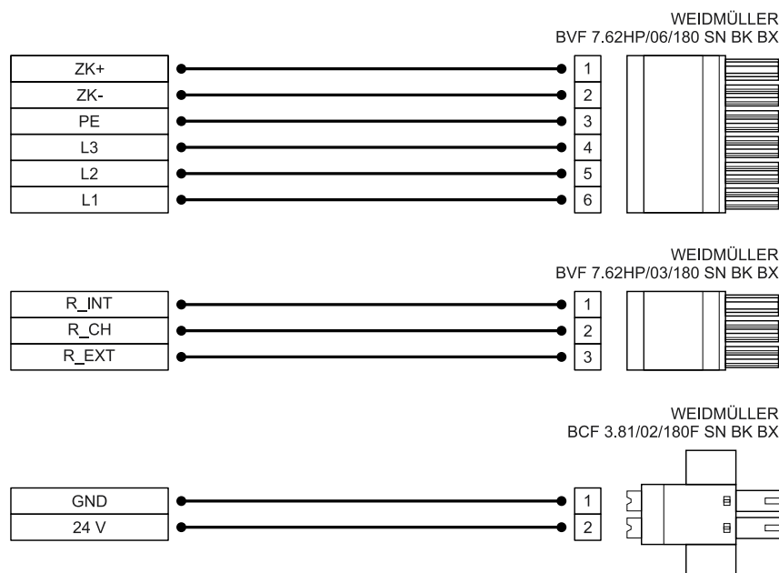
Abbildung 14: Steckerbelegung „Versorgungsspannung [X9], [X9A], [X9B]“
