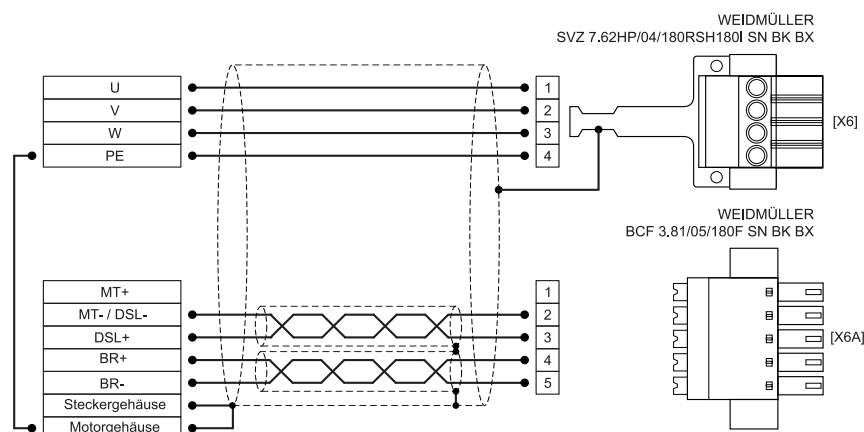
Abbildung 18: Steckerbelegung „Motor mit HIPERFACE DSL® [X6]“
