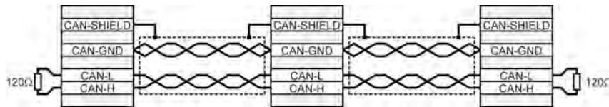
Abbildung 27: Verkabelungsbeispiel für CAN-Bus
