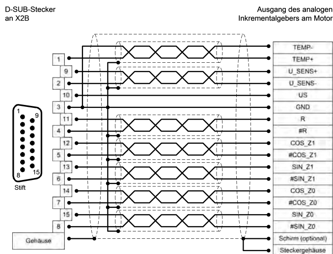
Abbildung 21: Steckerbelegung „Analoge Inkrementalgeber [X2B]“
