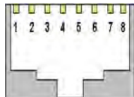
Abbildung 26: Steckerbelegung Netzwerkanschluss
