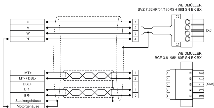
Abbildung 17: Steckerbelegung „Motor mit Motortemperatur-Sensor [X6]“
