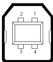
Abbildung 24: Steckerbelegung USB-Anschluss
