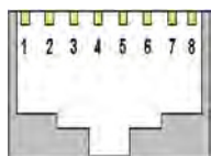
Abbildung 25: Steckerbelegung Netzwerkanschluss
