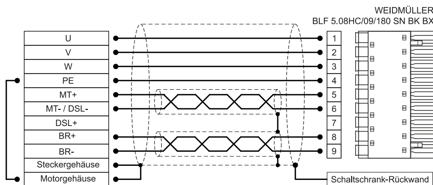
Abbildung 15: Steckerbelegung „Motor mit Motortemperatur-Sensor [X6]“
