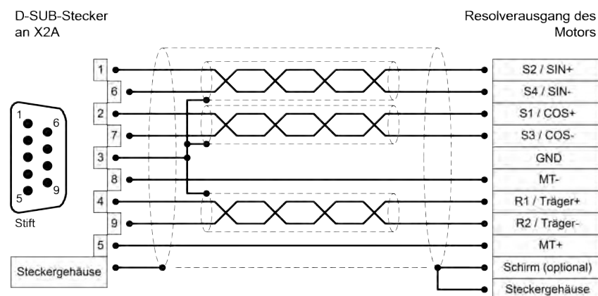
Abbildung 19: Steckerbelegung: Resolveranschluss [X2A]
