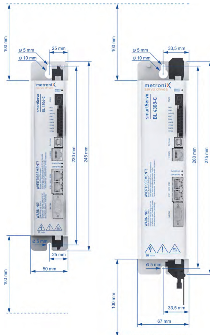
Abbildung 5: Servoregler BL 4100-C (links) und BL 4300-C (rechts)
