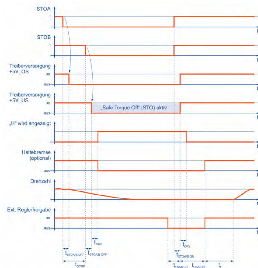
Abbildung 9: Zeitverhalten beim Aktivieren der Sicherheitsfunktion STO mit Wiederanlauf
