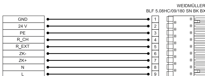
Abbildung 12: Steckerbelegung „Versorgungsspannung [X9]“
