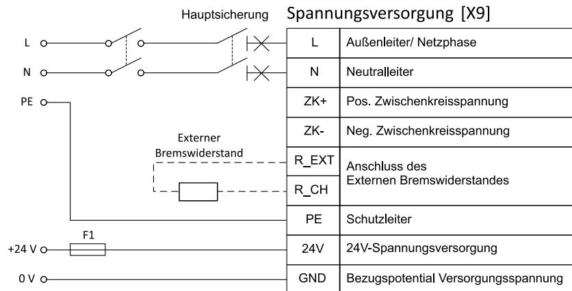
Abbildung 11: Anschluss eines BL 4100-C an die Versorgungsspannung [X9]
