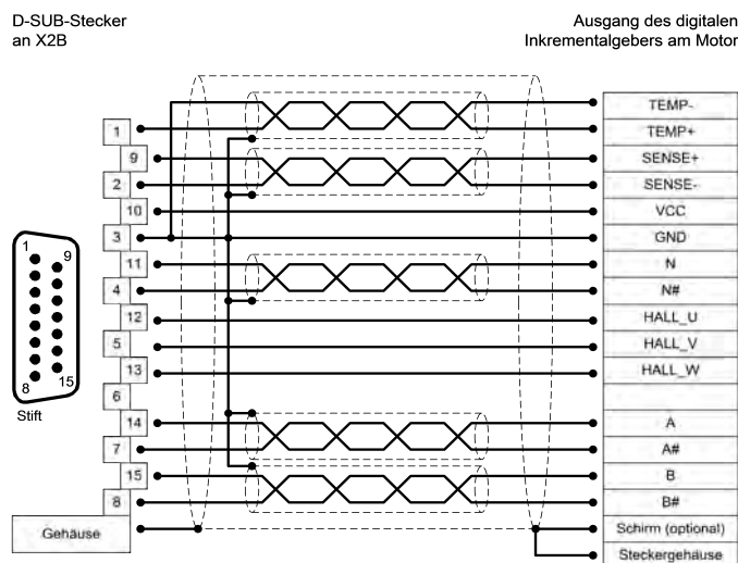
Abbildung 23: Steckerbelegung „Digitale Inkrementalgeber (RS422) [X2B]“
