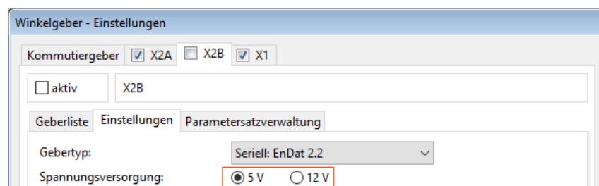
Abbildung 20: Winkelgeber-Einstellungen: Parametrierung der Versorgungsspannung
