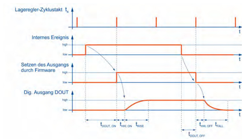
Abbildung 7: Mechanismus der Filterzeit bei digitalen Ausgängen
