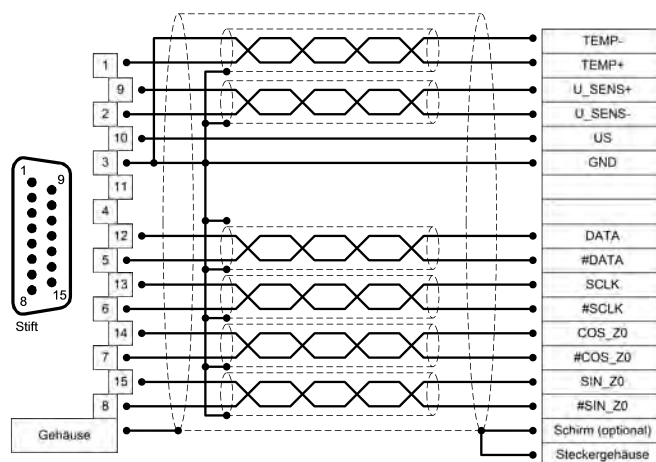
Abbildung 22: Steckerbelegung „Inkrementalgeber mit serieller Schnittstelle [X2B]“
