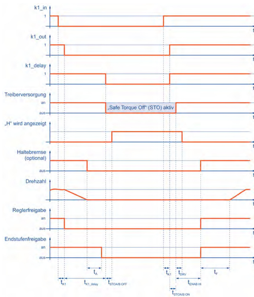
Abbildung 10: Zeitverhalten beim Aktivieren der Sicherheitsfunktion SS1 (externe Beschaltung) mit Wiederanlauf
