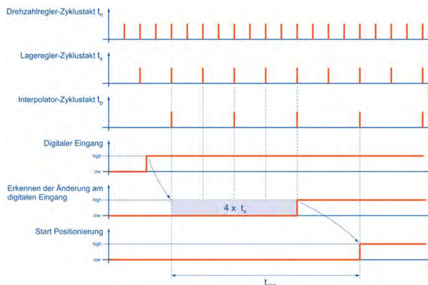
Abbildung 6: Mechanismus der Filterzeit bei digitalen Eingängen
