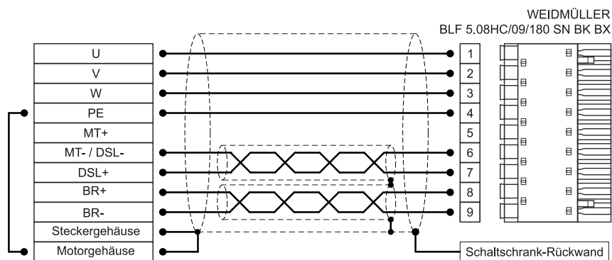
Abbildung 16: Steckerbelegung „Motor mit HIPERFACE DSL® [X6]“
