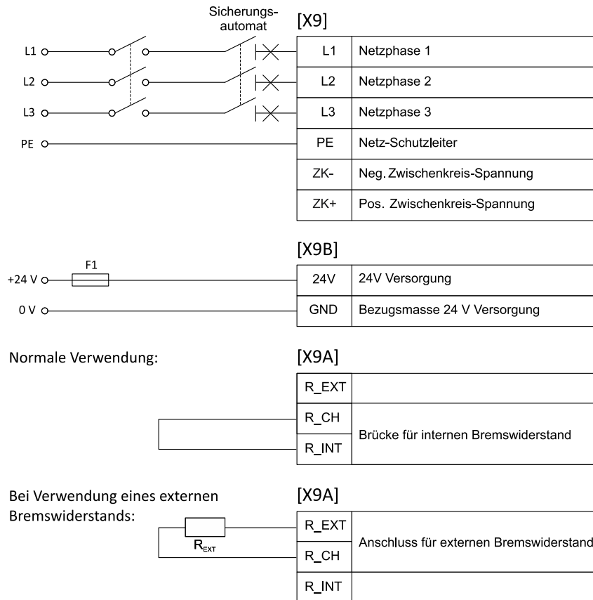
Abbildung 13: Anschluss eines BL 4300-C an die Versorgungsspannung [X9]
