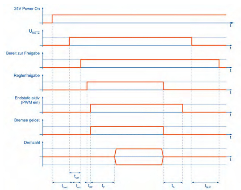
Abbildung 8: Timingdiagramm des Servoreglers
