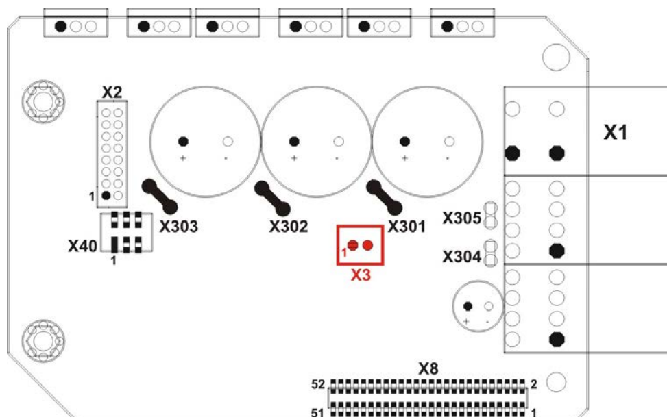
Abbildung 28: Position und Anschluss Haltebremse
