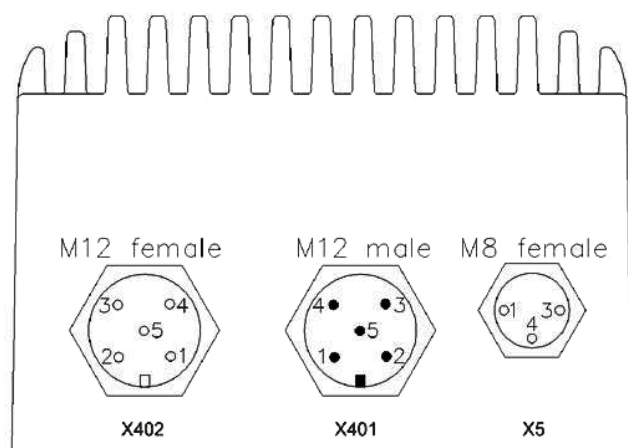
Abbildung 32: Position und Anschluss RS232 Schnittstelle
