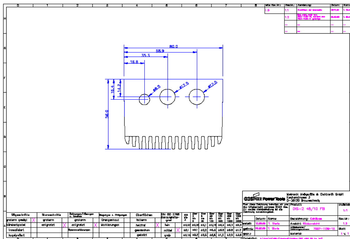
Abbildung 19: Gehäuseabmessungen
