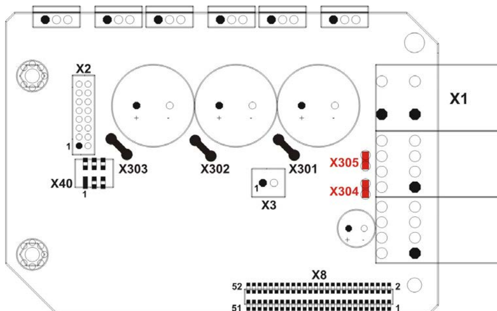
Abbildung 29: Position und Anschluss Bremswiderstand
