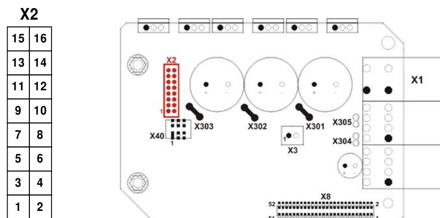
Abbildung 27: Position und Anschluss Winkelgeber
