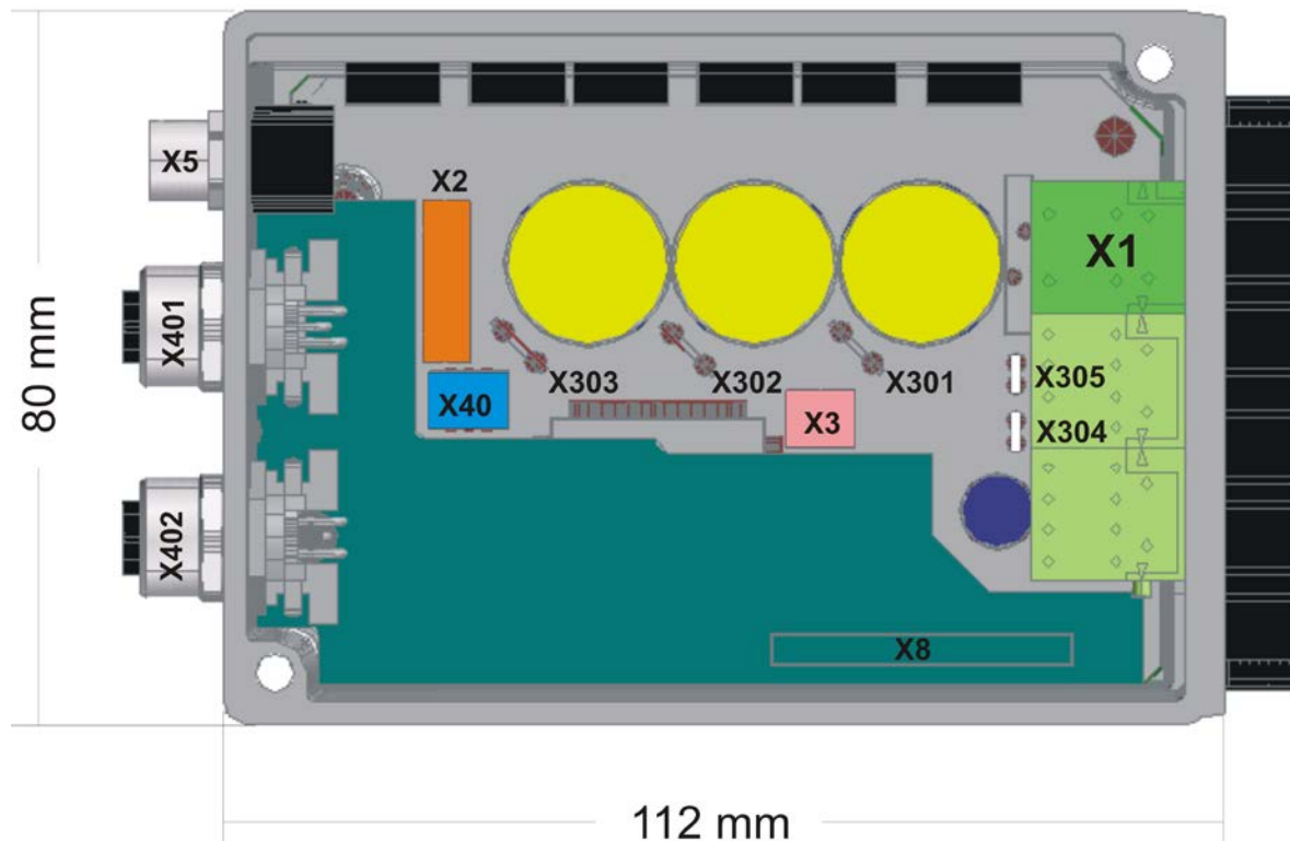
Abbildung 18: Anordnung Steckverbinder DIS-2 48/10 FB FS STO – Draufsicht des Gerätes
