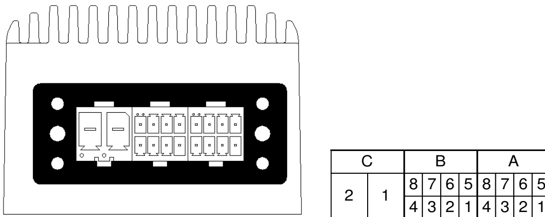
Abbildung 25: Anschluss und Pin-Nummerierung [X1]
